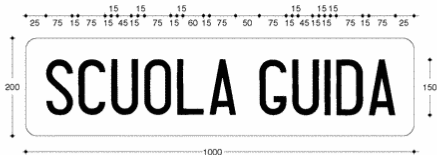
Figura IV 5 Art. 334 CONTRASSEGNO ANTERIORE E POSTERIORE PER I VEICOLI DELLE CATEGORIE M2-M3-N2-N3 CON- TRASSEGNO POSTERIORE PER VEICOLI DELLE CATEGORIE 03-04 (dimensioni in millimetri)
